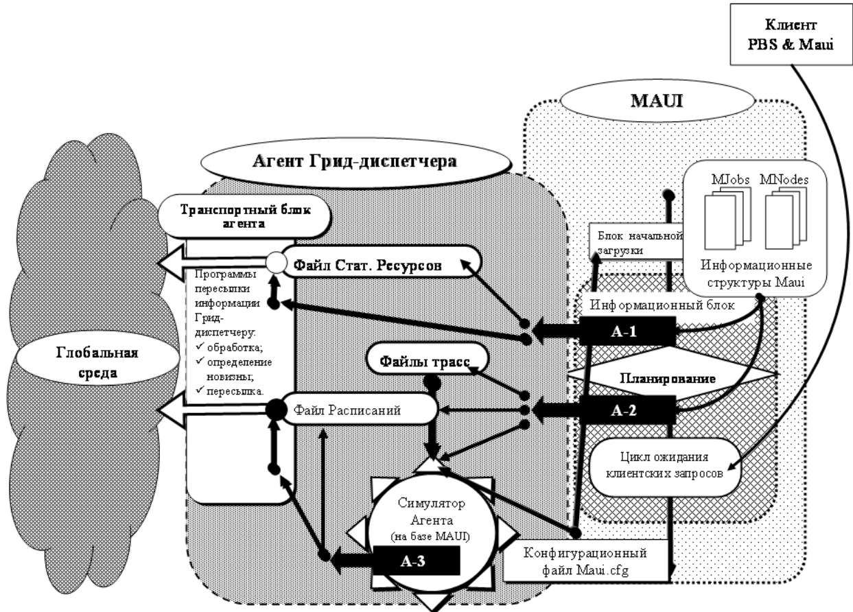
Рисунок 2. Схема взаимодействий между компонентами Maui и Агента GrAS
